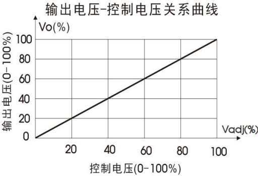
(注: 100% Vadj 等于 5.0VDC (Typ.)) 图 3 输出电压与控制电压关系曲线
