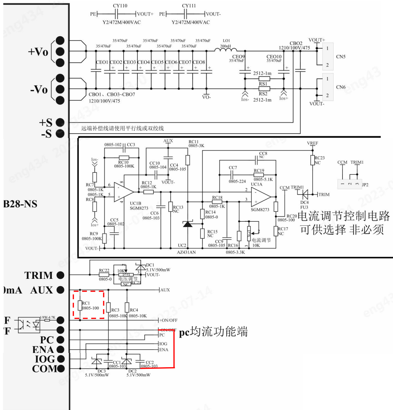
图 4 遥控功能屏蔽连接示意图
