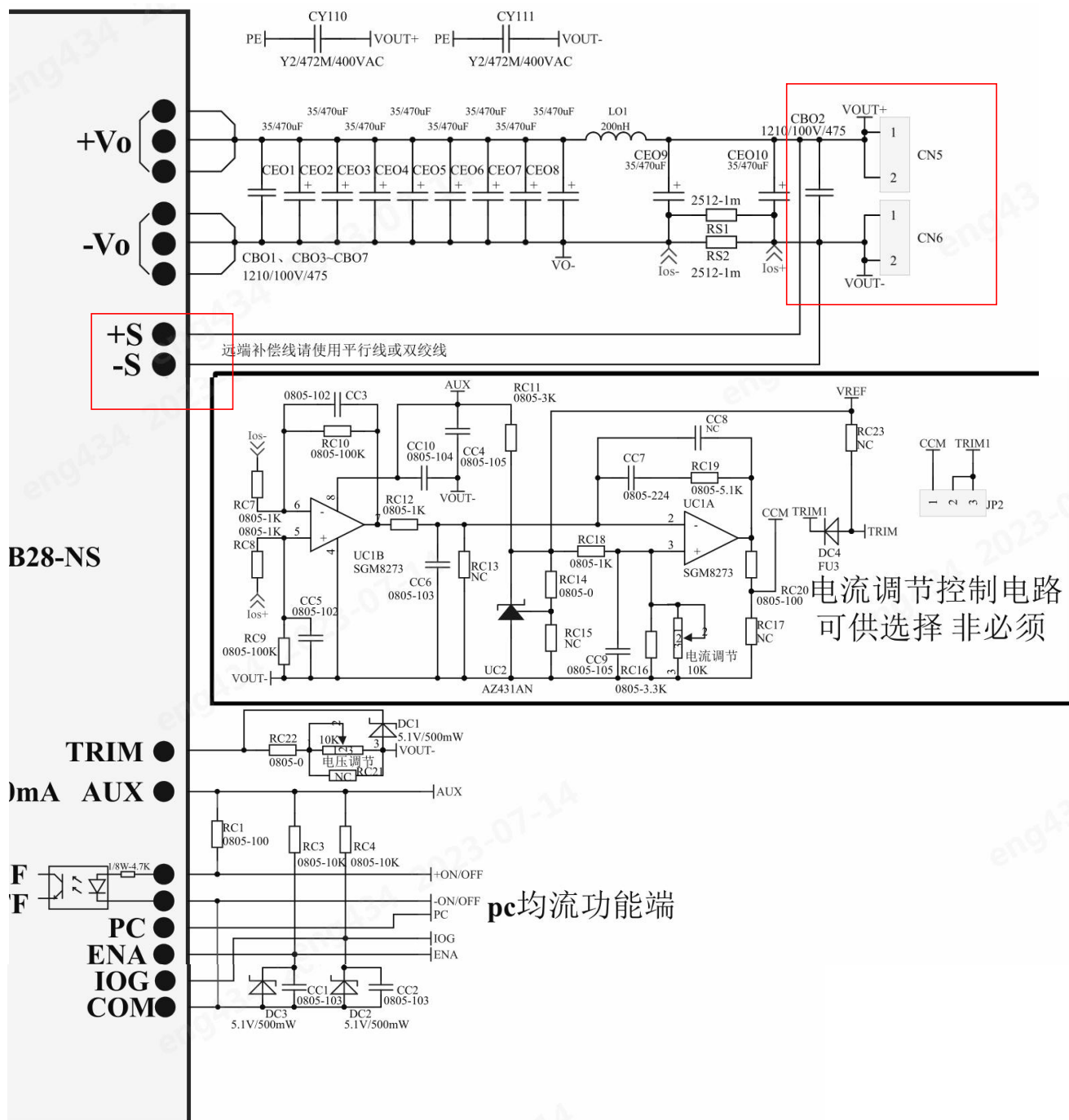
图 2 远端补偿接线示意图
