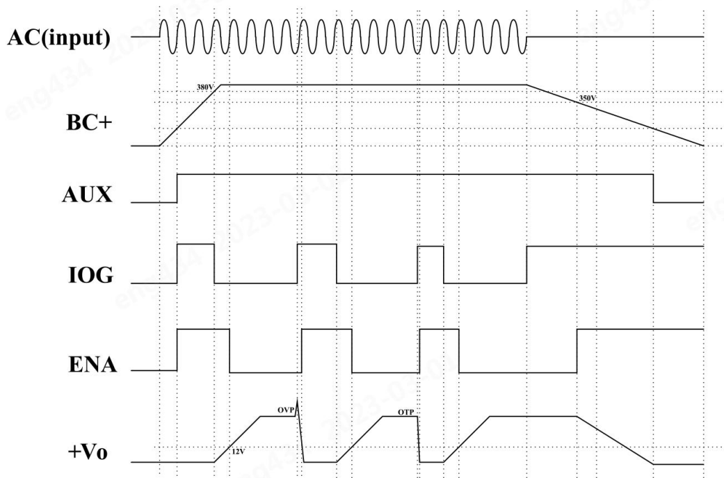
电路时序图
