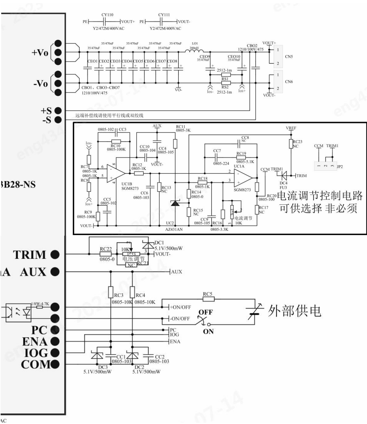
图 5 遥控开关连接示意图
