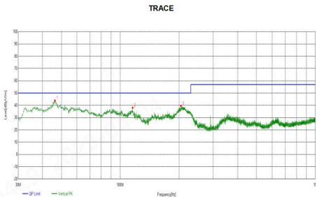
垂直波形及读点
