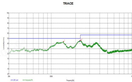
水平波形及读点
