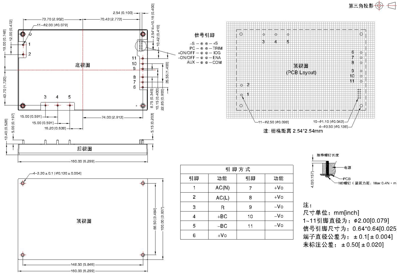
图 7 制造数据/尺寸图
