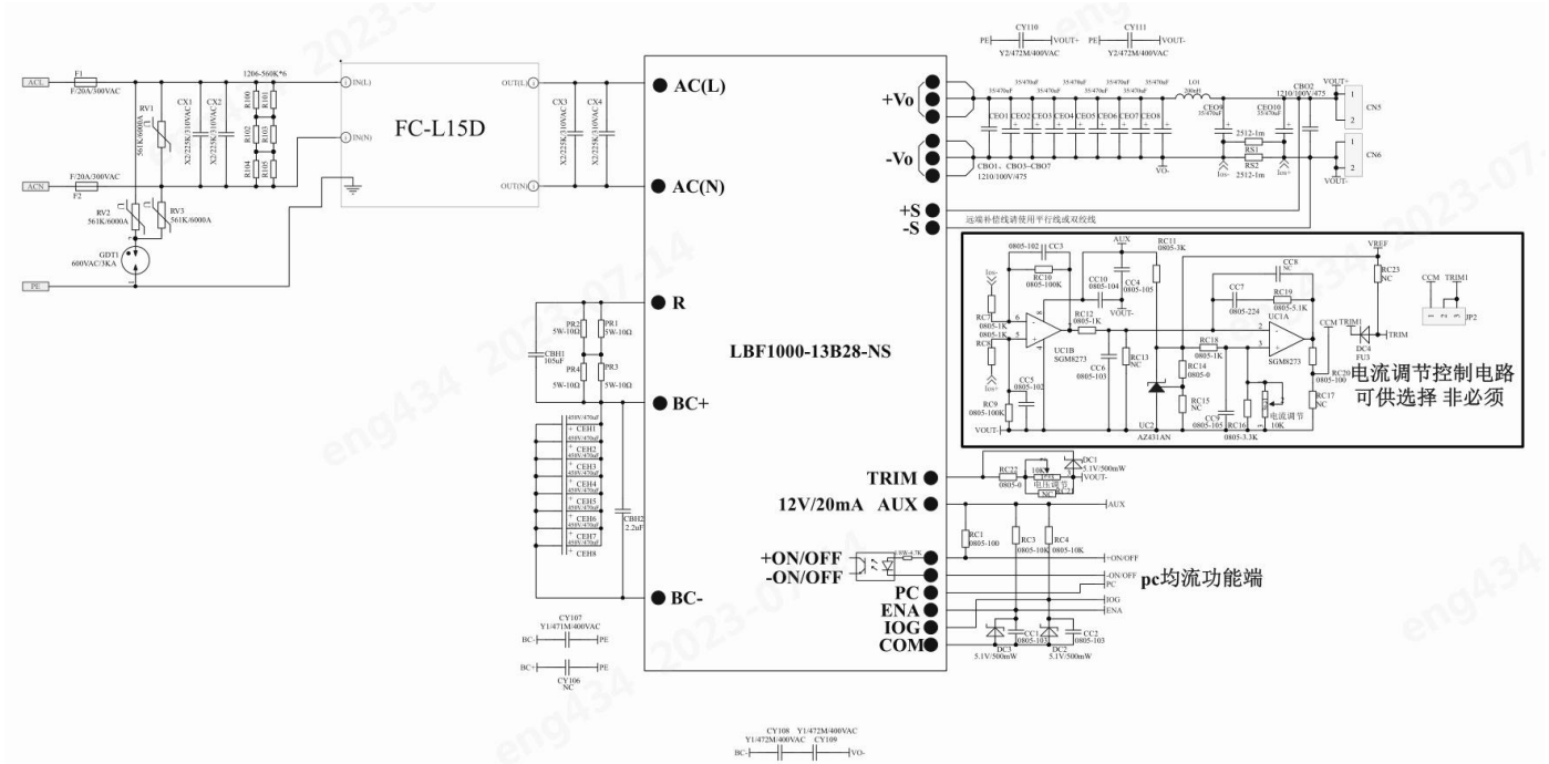
推荐外围电路 1
