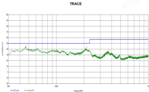
垂直波形及读点
