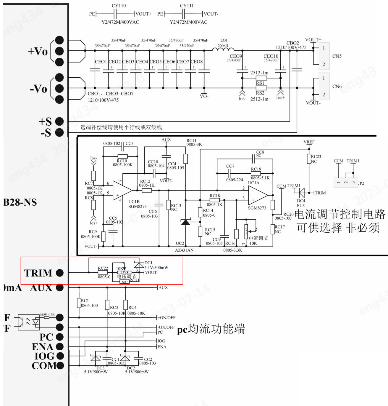
图 3 输出电压调节连接示意图
