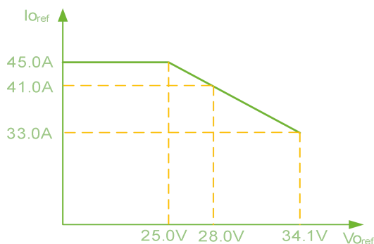
图 5 输出电压给定值与恒流点之间关系图
