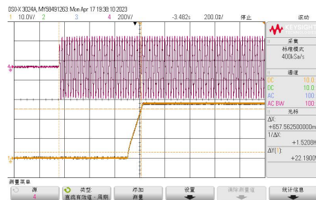
Vin=230VAC 满载启机（启机延迟 657ms）
