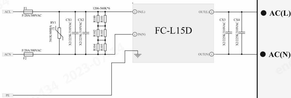
推荐外围电路 3 (EMC 部分)
